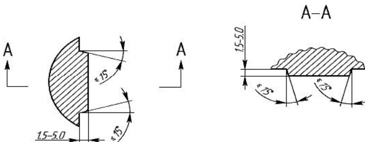
Рисунок 7 - Скосы краев и впадин
