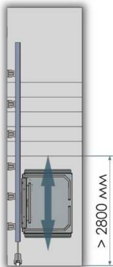
Платформа проходная (нижняя площадка более 2800 мм)
